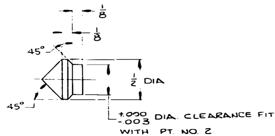
9 END CAP SCALE: 2x
